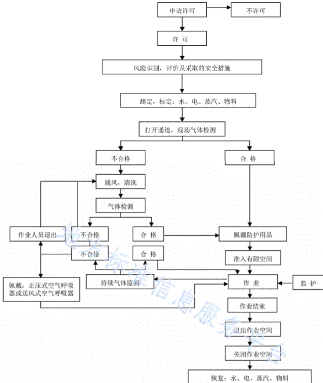
图A.1 进入有限空间作业流程
