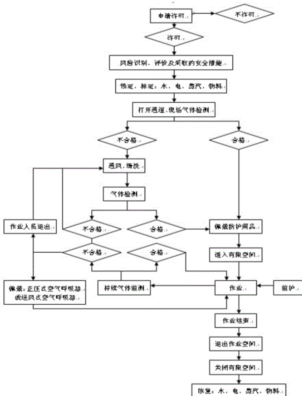
图 B.1 进入有限空间危险作业流程
