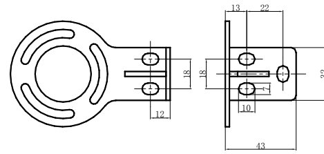
图 2 墙壁方式尺寸图
