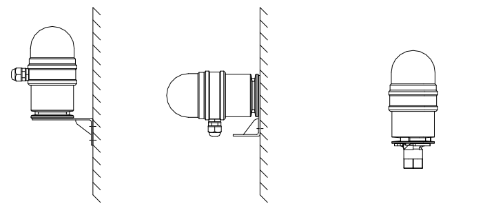
图 4 安装方式图
