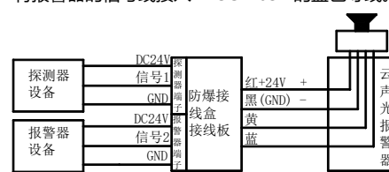
图 3 带防爆接线盒接线
