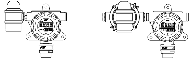
图 2 安装示意图
