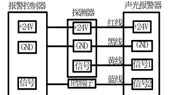
图 4 无防爆接线盒接线
